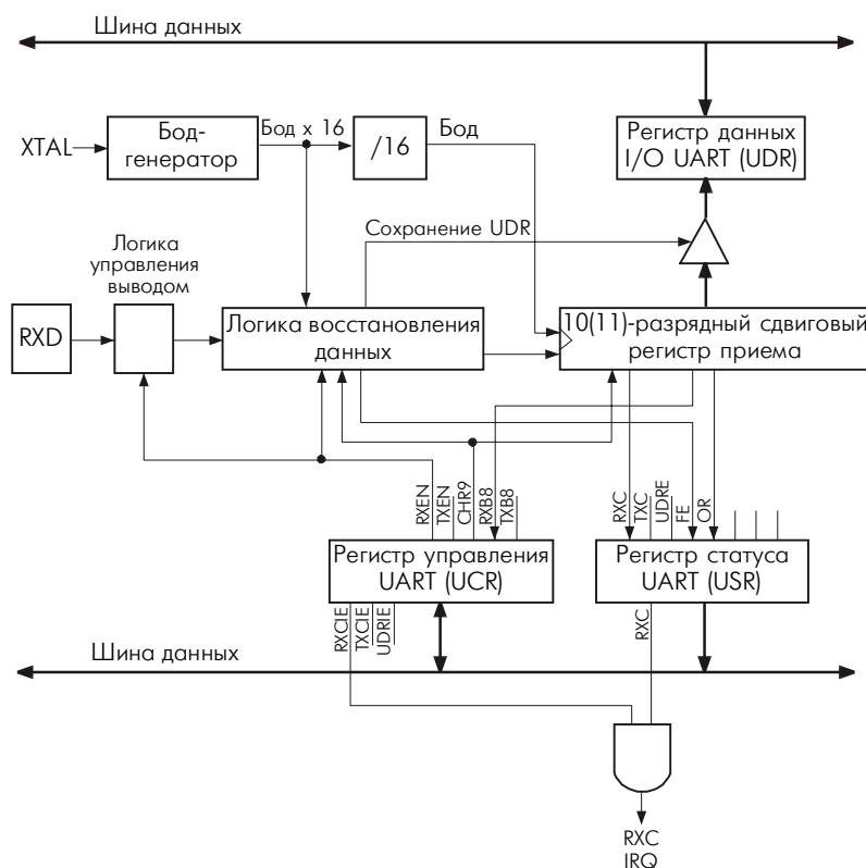
Рис. 43 Приемник UART.
