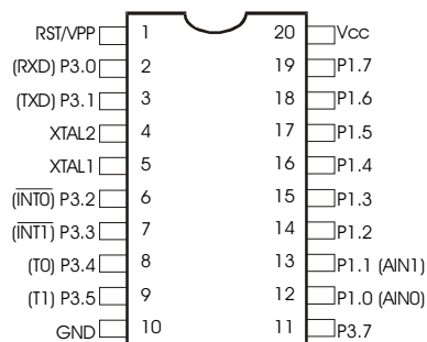
Корпус PDIP/SOIC
