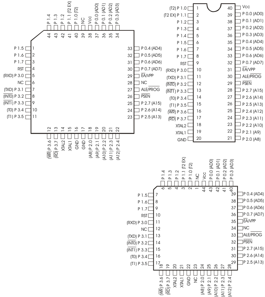
Корпус PLCC/LCC
