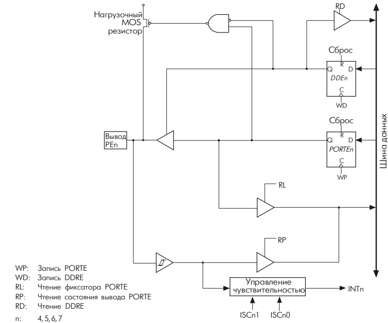
Рис. 65 Схема организации выводов порта E (выводы с PE4 по PE7)
