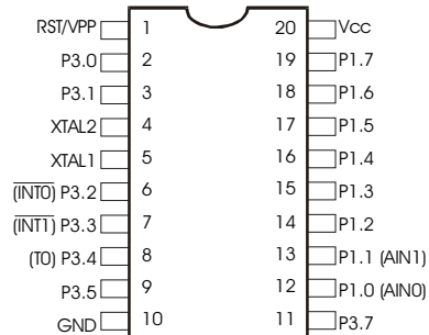
Корпус PDIP/SOIC
