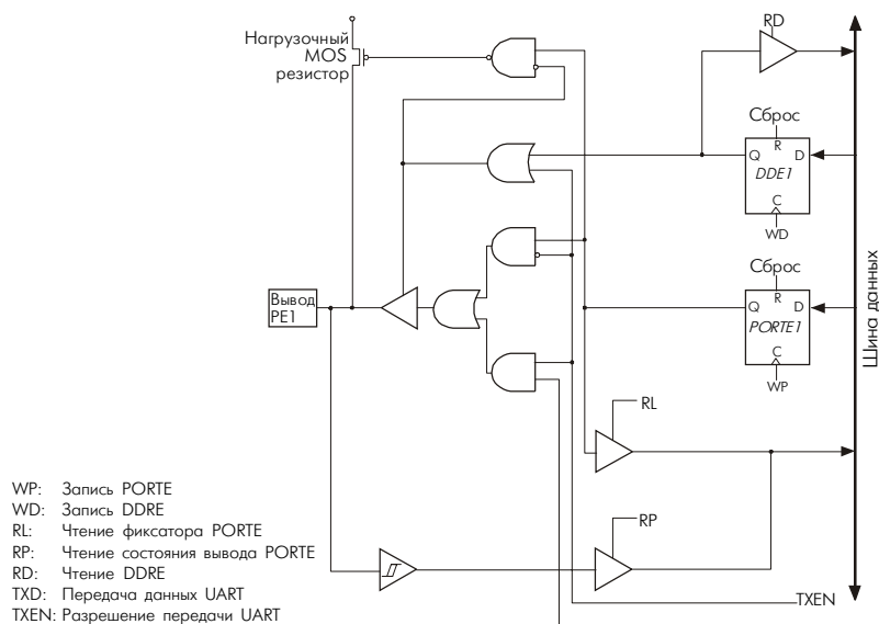
Рис. 62 Схема организации вывода порта Е (вывод PE1)
